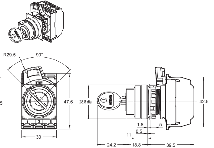
A22NK-2B□-01□A-P
