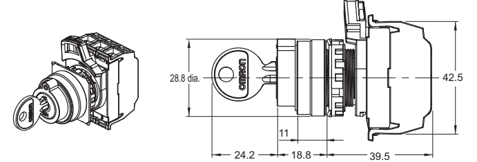
A22NK-3M□-01□A-P
