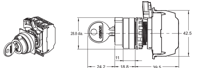
A22NK-3B□-01□A-P
