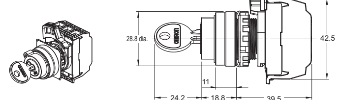
A22NK-2M□-01□A-P
