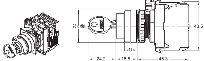
A22NK-2M□-01□A-G
